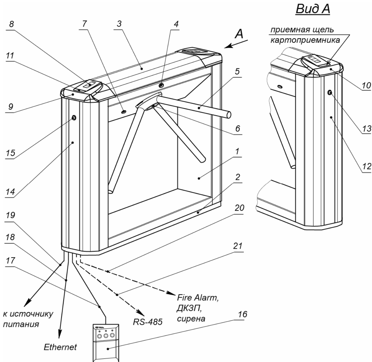
Рисунок 1. Устройство ЭП
